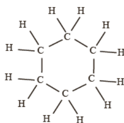
سیکلوهگزان
