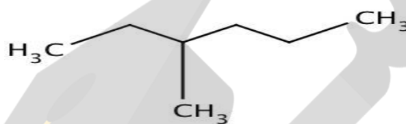
۳- متیل هگزان
