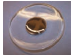
شکل ۲-۹ الف) پخش آب روی سطح شیشه (ب) قطره‌ای شدن جیوه روی سطح شیشه
