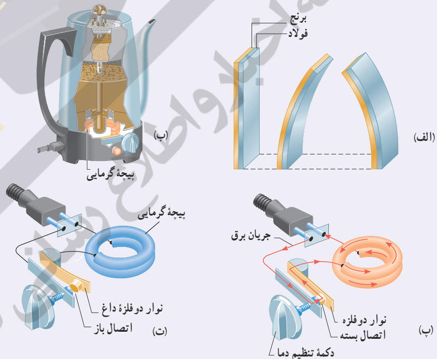
شکل ۱۱-۴ الف تیغه دوفلزه با تغییر دما در جهت‌های مختلفی خم می‌شود، (ب) دماپا در یک کتری برقی، (پ) با برقرار شدن جریان الکتریکی، نوار دوفلزه گرم می‌شود. (ت) سپس نوار خم شده و اتصال را قطع می‌کند.
