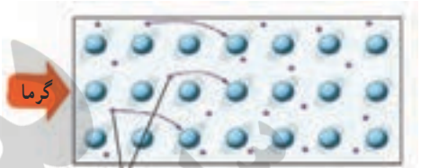
الکترون‌های آزاد
