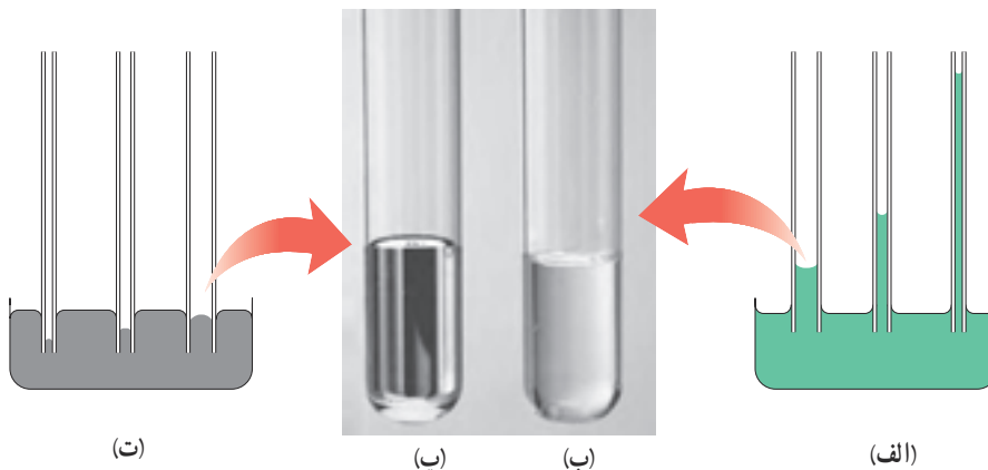
شکل ۱-۲ الف و ب) اثر موینگی برای آب (ب) و (ت) اثر موینگی برای جیوه
