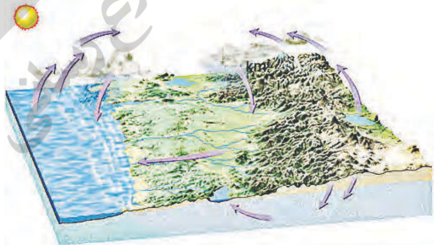
شکل ۱۳- چرخه آب
