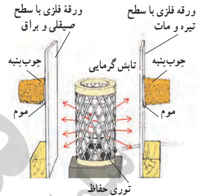
شکل ۱۰ - جذب تابش گرمایی
